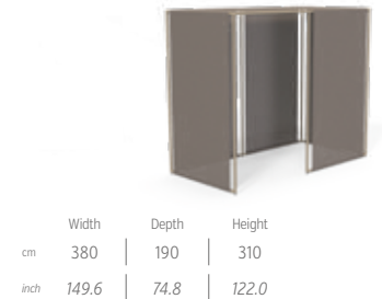
MODULE C1 380X190 H310 / CODE: SKYMODC1
